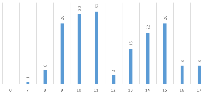
2025 RÉPARTITION DES ESSAIS MOTEURS PAR TRANCHES HORAIRES
